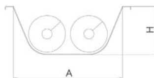
ESTRATTORI A DOPPIA COCLEA mod. AG/W DOUBLE SCREW EXTRACTORS
