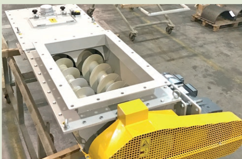
Estrattori a doppia coclea in acciaio INOX Double Stainless-Steel Screw Extractor Extracteurs à double vis en acier INOX
