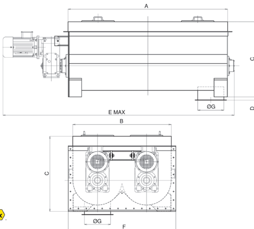
Miscelatore MA/2 – Lt. 4000 con tramoggia di scarico rapido. Mixer MA/2 – Lt. 4000 with under hopper for fast discharge.
